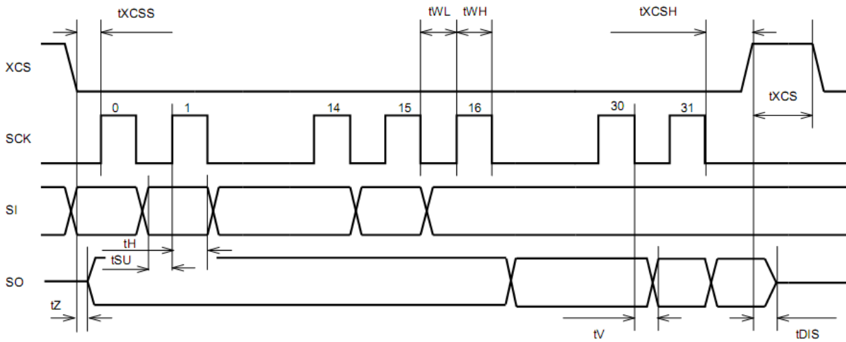
图 9: SPI 时序图
